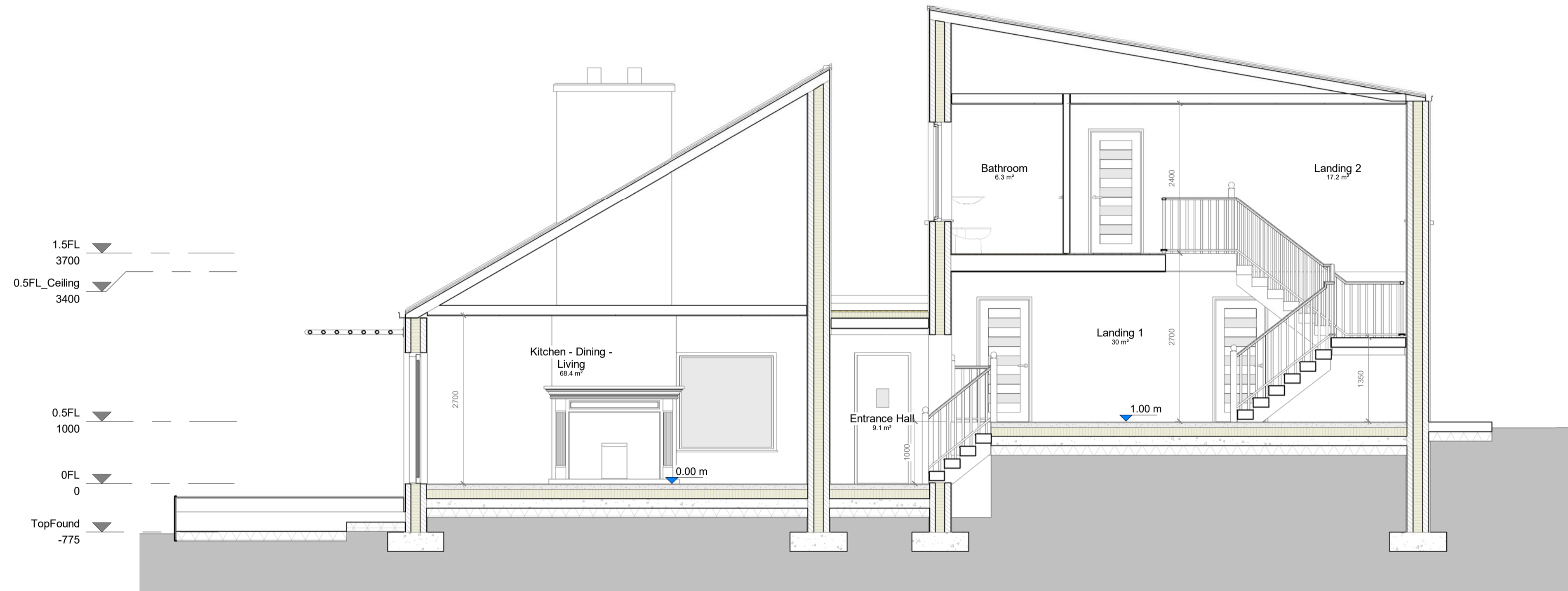
Section 1 1 : 50
